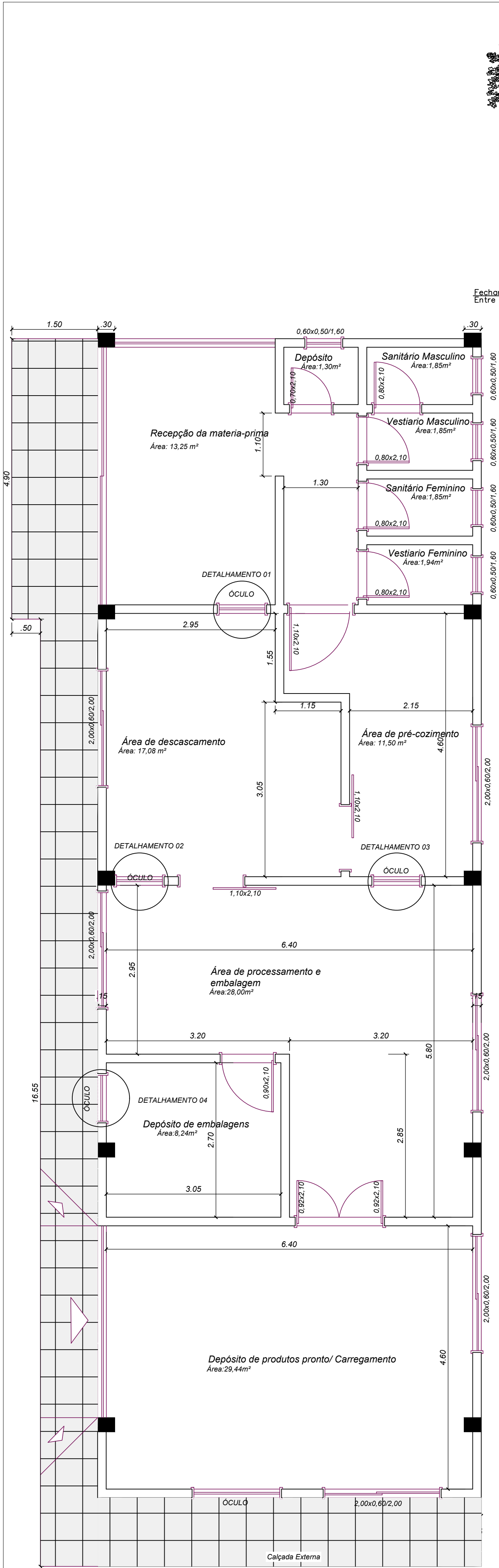
01 PLANTA BAIXA-TÉCNICA ESCALA: 1/50
