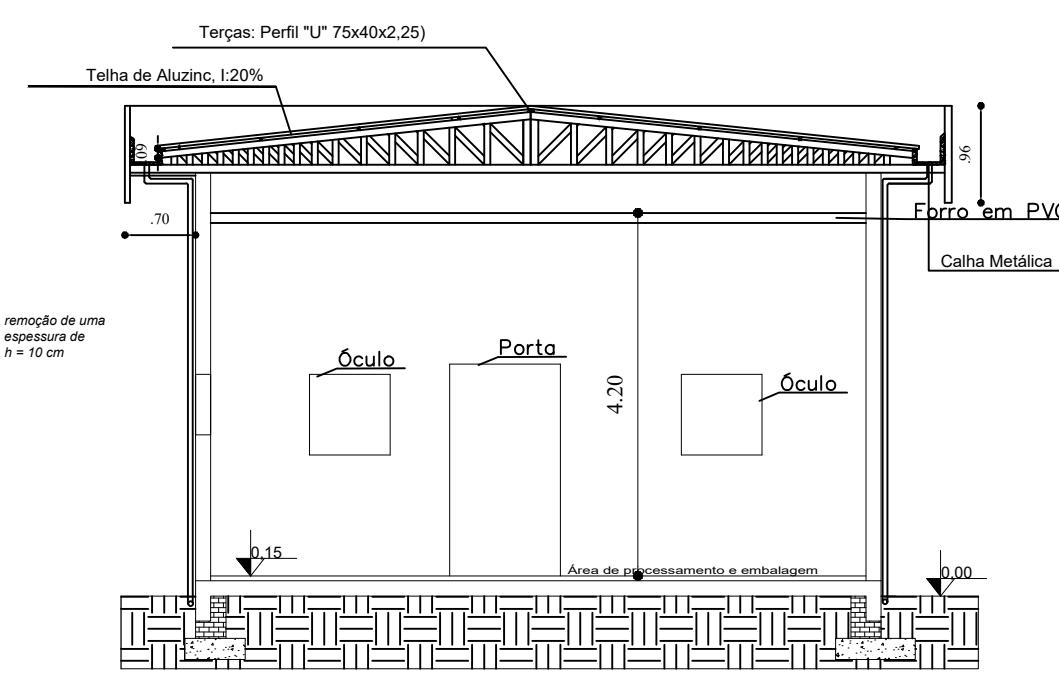
04 CORTE B-B ESCALA: 1/75
